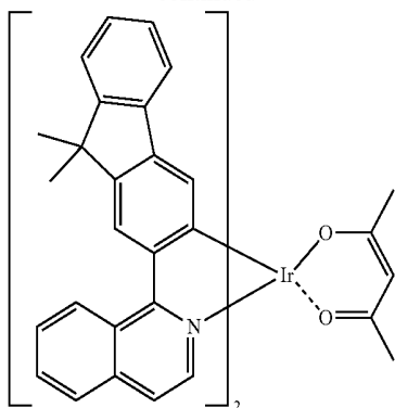
Ir(fliq) 2 (acac)
