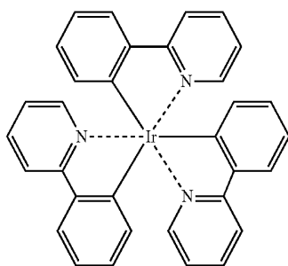
Ir(ppy) 3
