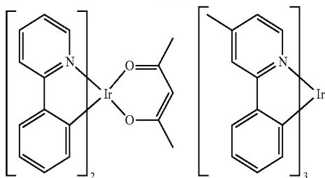
Ir(ppy) 2 (acac)
