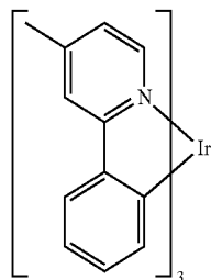
Ir(mppy) 3
