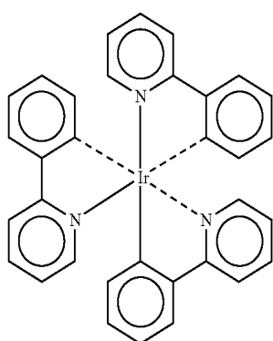
Ir(ppy) 3
